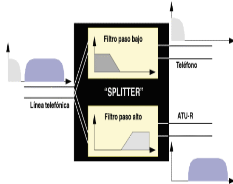
Funcionamiento del "splitter"
