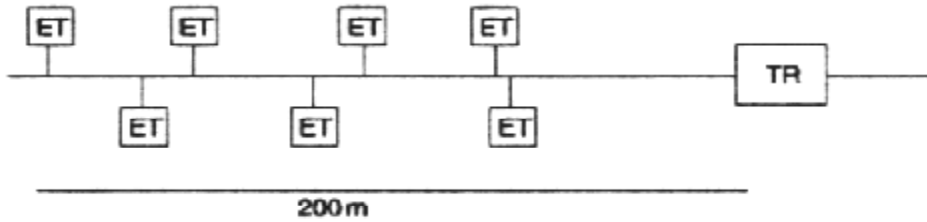
Bus corto
