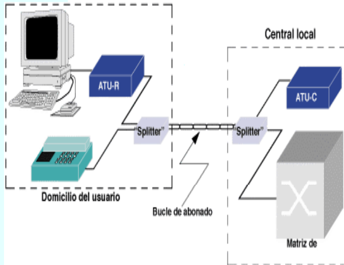
Enlace ADSL
