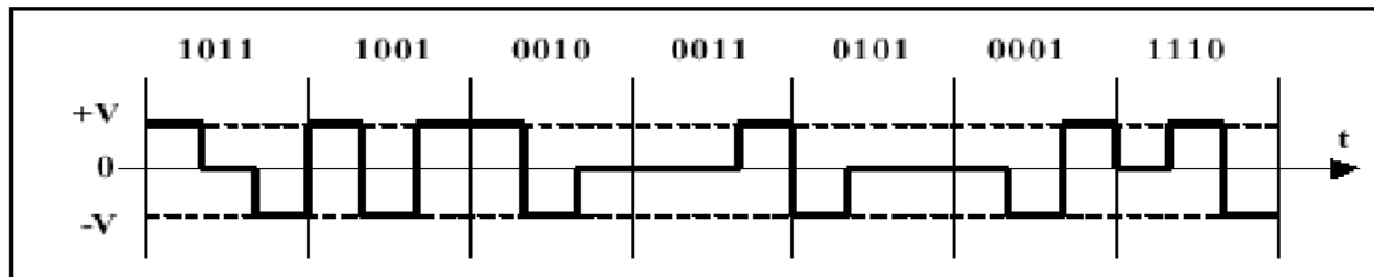
Ejemplo de codificación 4B3T.
