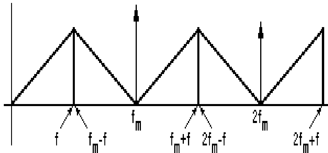
ESPECTRO
