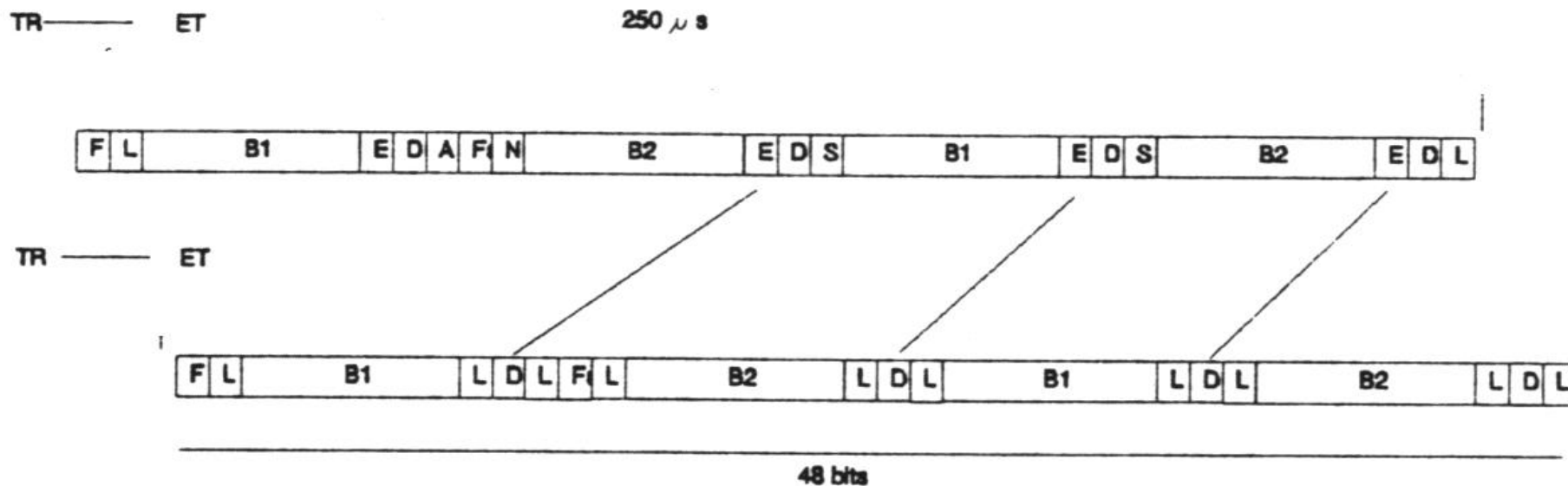
Estructura de trama en acceso básico
