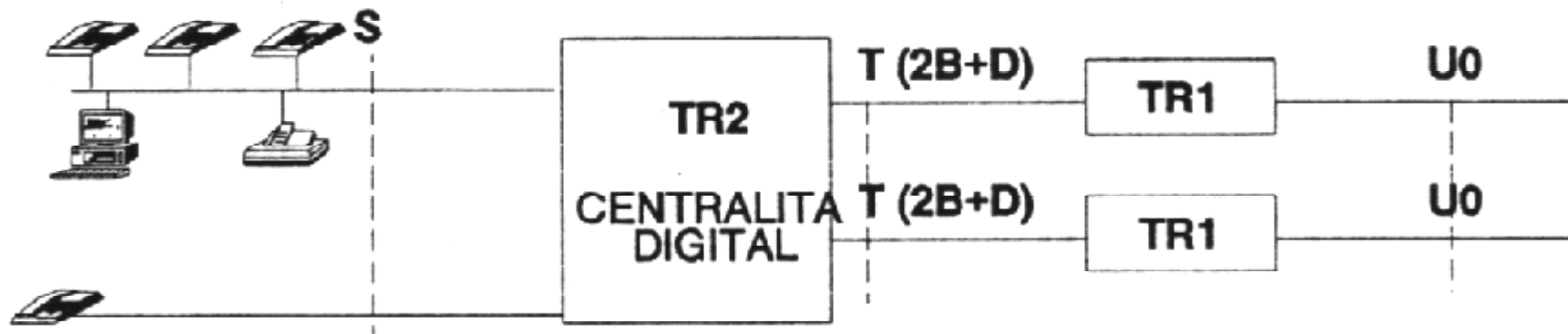
Interconexión a través de varios Accesos Básicos
